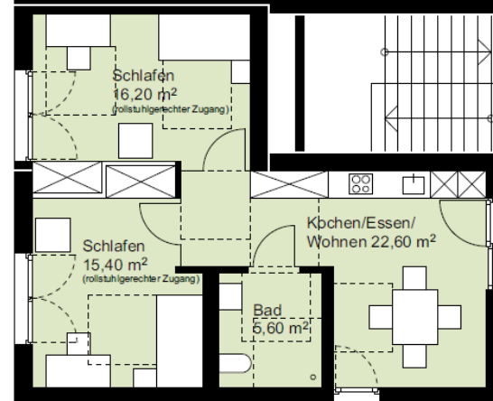
2-Raum-Wohnung 59,80 m 2
